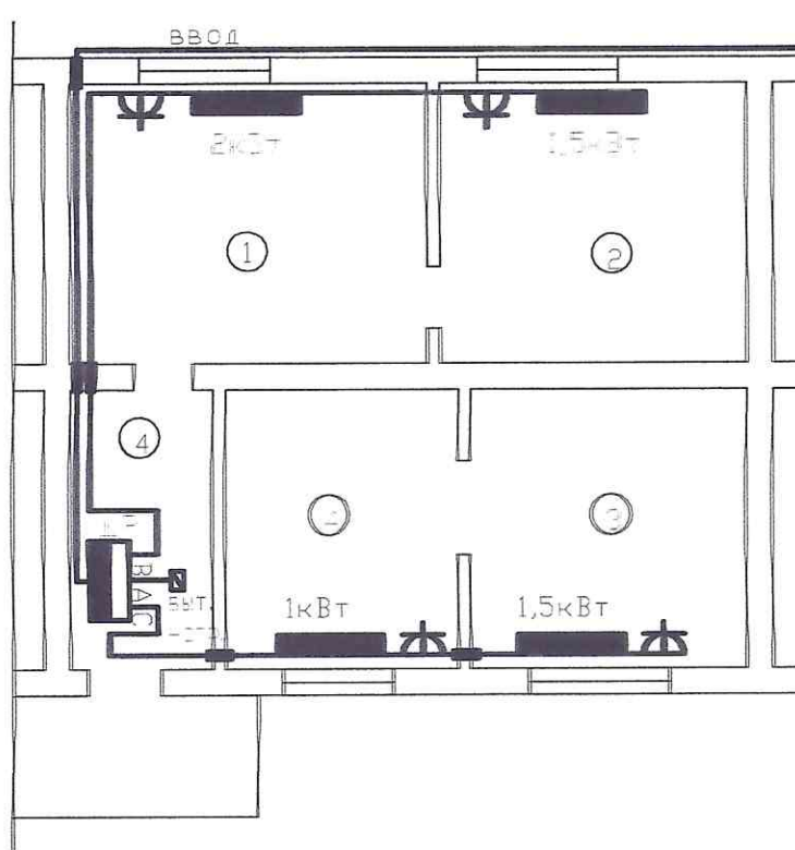
Экспликация помещения
